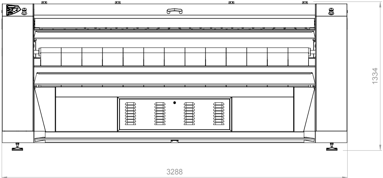
VORDERANSICHT
