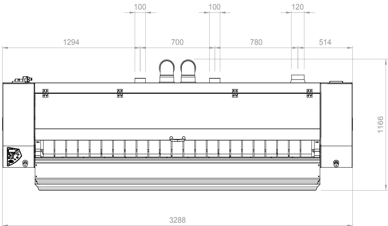
DRAUFSICHT
